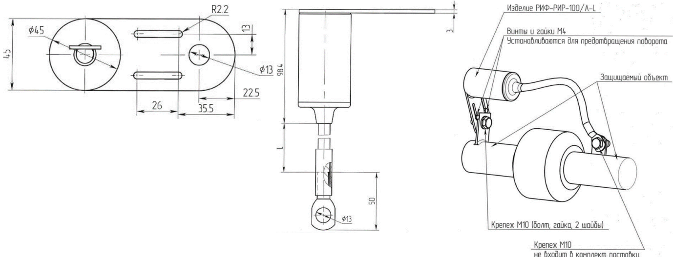
Пример монтажа
